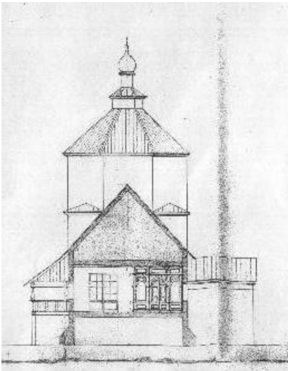
План деревянного храма во имя Всех Святых (бывшего Покровского), г. Меленки
